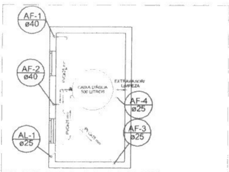
03 Planta Baixa Laje da Caixa D'água ESCALA 1:50
