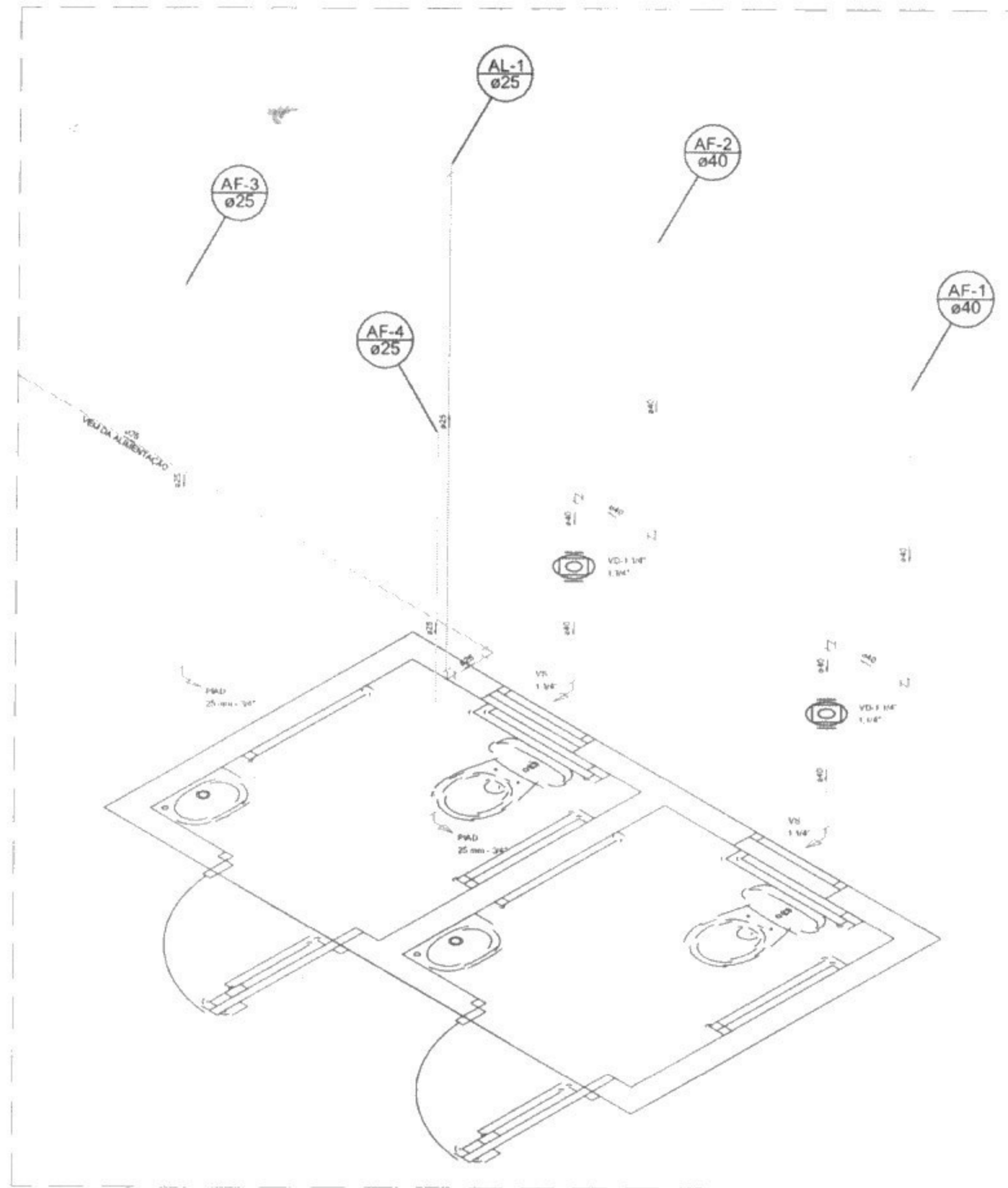
02 Isométrico dos Banheiros Acessíveis ESCALA 1:25
